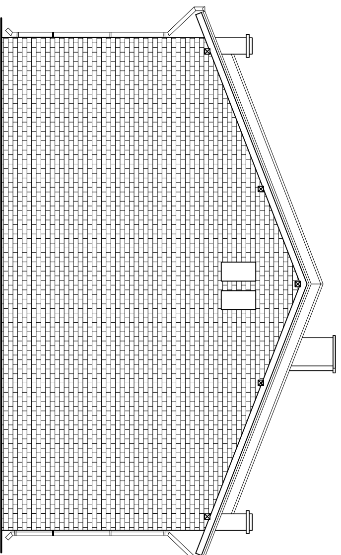
Elewacja północna
