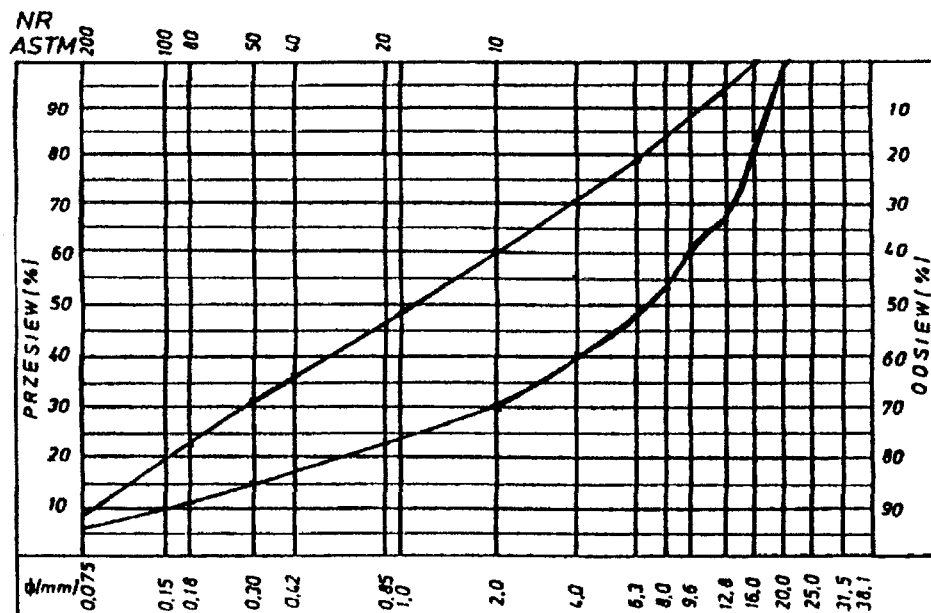
Rys. 1. Krzywe graniczne uziarnienia mieszanki mineralnej 0÷20 mm do warstwy ościeralnej z betonu asfaltowego dla KR 1-2
