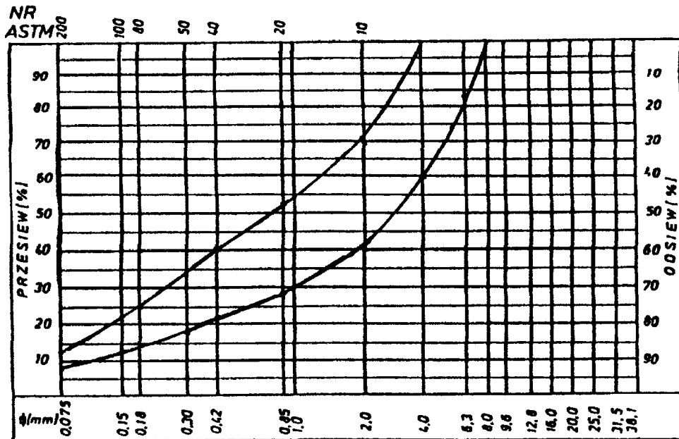
Rys. 3. Krzywe graniczne uziarnienia mieszanki mineralnej 0÷8, 0÷6,3 mm do warstwy cieżarnej z betonu asfaltowego dla KR 1-2
