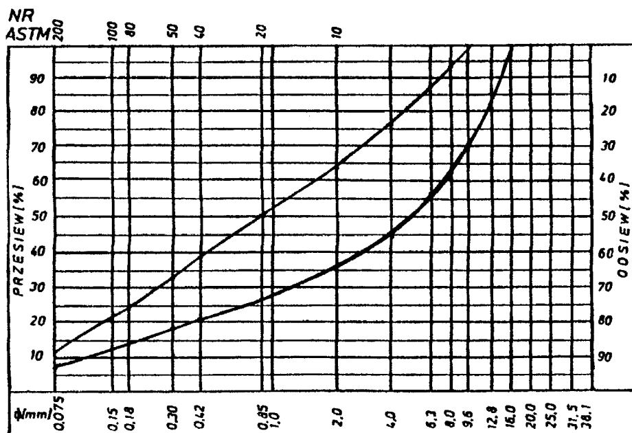
Rys. 2. Krzywe graniczne uziarnienia mieszanki mineralnej 0÷16, 0÷12,8 mm do warstwy ościeralnej z betonu asfaltowego dla KR 1-2
