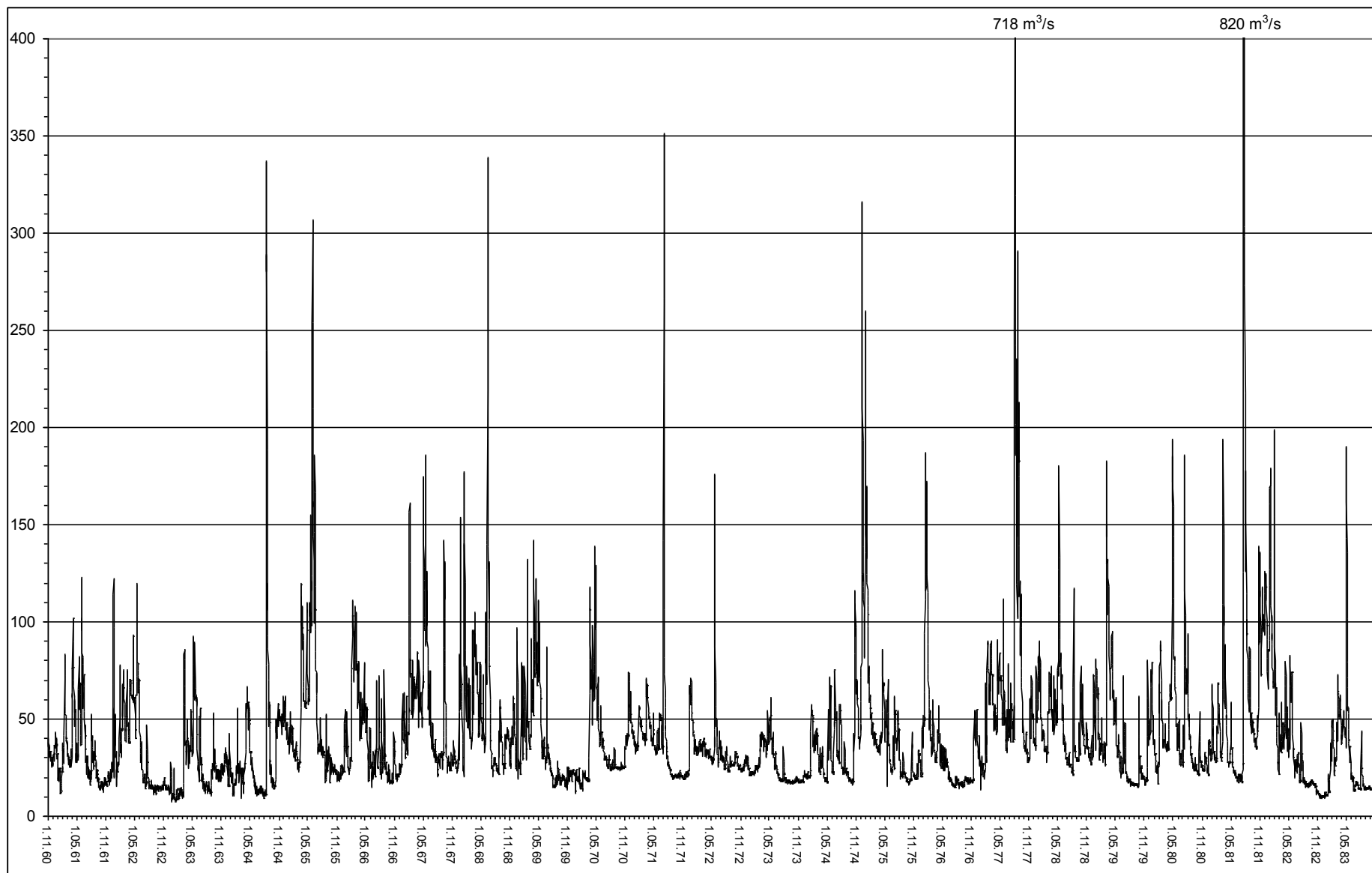
Rys. 3. Hydrogram przepływów Bobru (w m 3 /s) na posterunku obserwacyjnym IMGW w Żaganiu (1.11.1960-1.11.1983).
