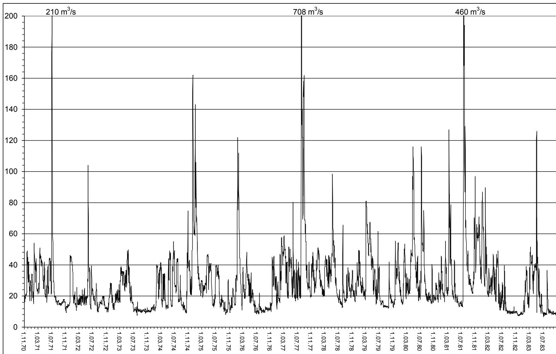
Rys. 2. Hydrogram przepływów Bobru (w \text{m}^3/\text{s} ) na posterunku obserwacyjnym IMGW w Szprotawie (1.11.1970-1.11.1983).
