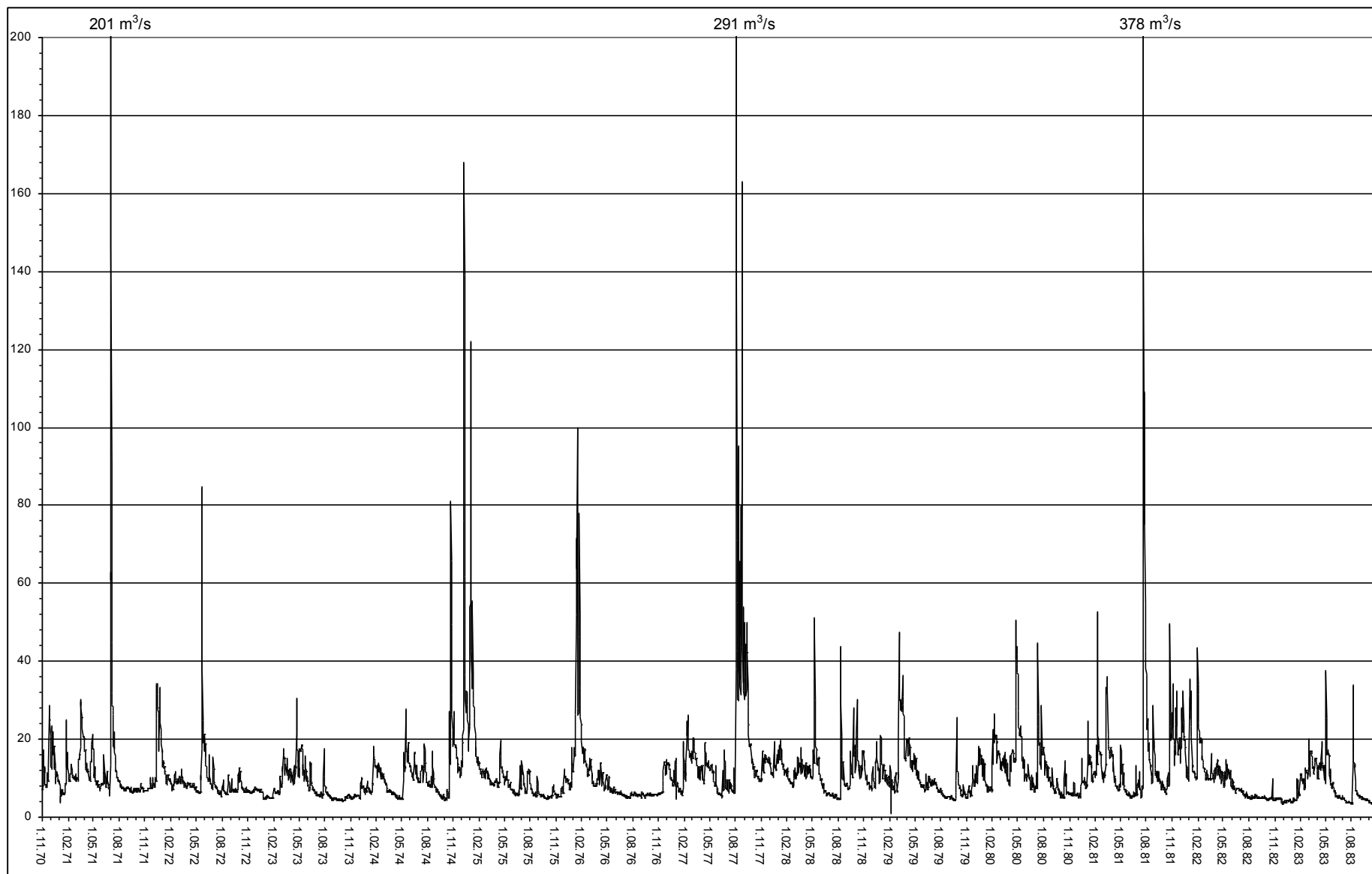
Rys. 4. Hydrogram przepływów Kwisy (w \text{m}^3/\text{s} ) na posterunku obserwacyjnym IMGW w Łozach (1.11.1970-1.11.1983).
